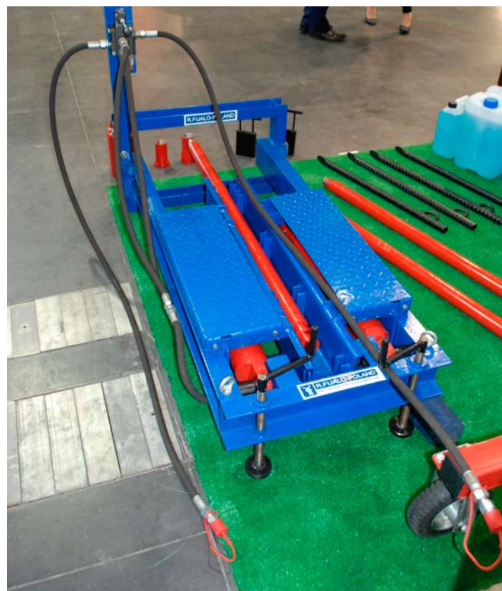
Hydrauliczna maszyna przeciskowa firmy R.Fijalo-Poland to ciekawa, a przy tym sporo tańsza alternatywa dla urządzeń przeciskowych typu „kret”.
